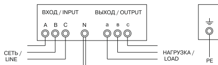
Рисунок 6 – Схема подключения СНИЗ-3 кВА
